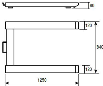
Dimensiones (mm)
