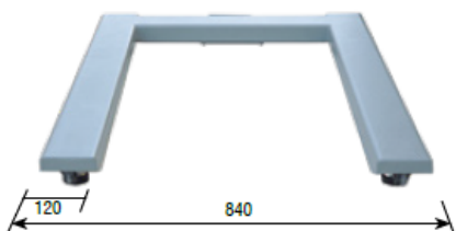
Dimensiones (mm)
